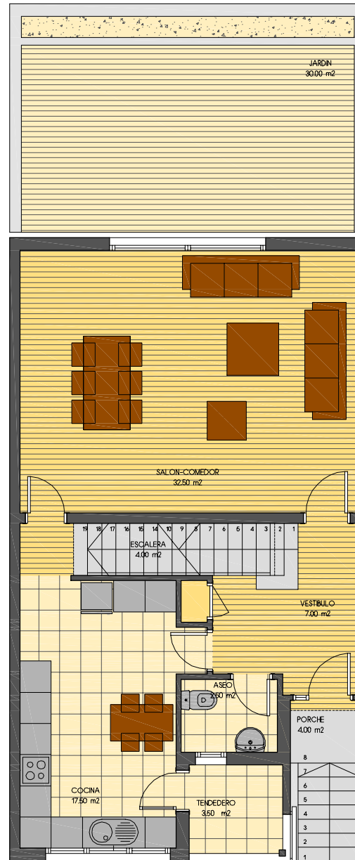
PLANTA BAJA
