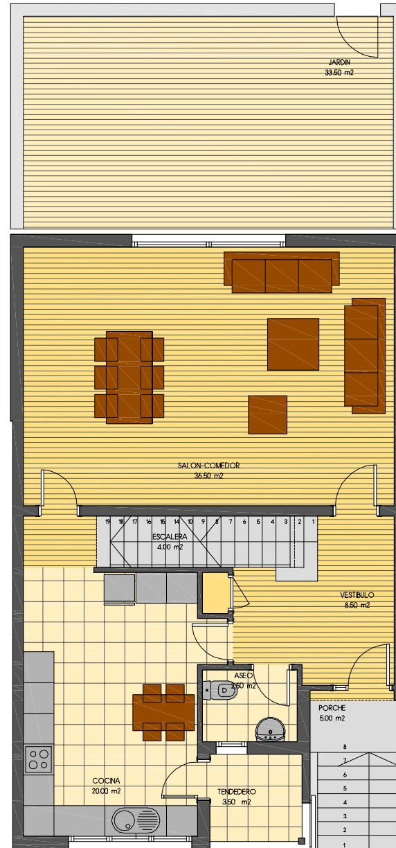
PLANTA BAJA
